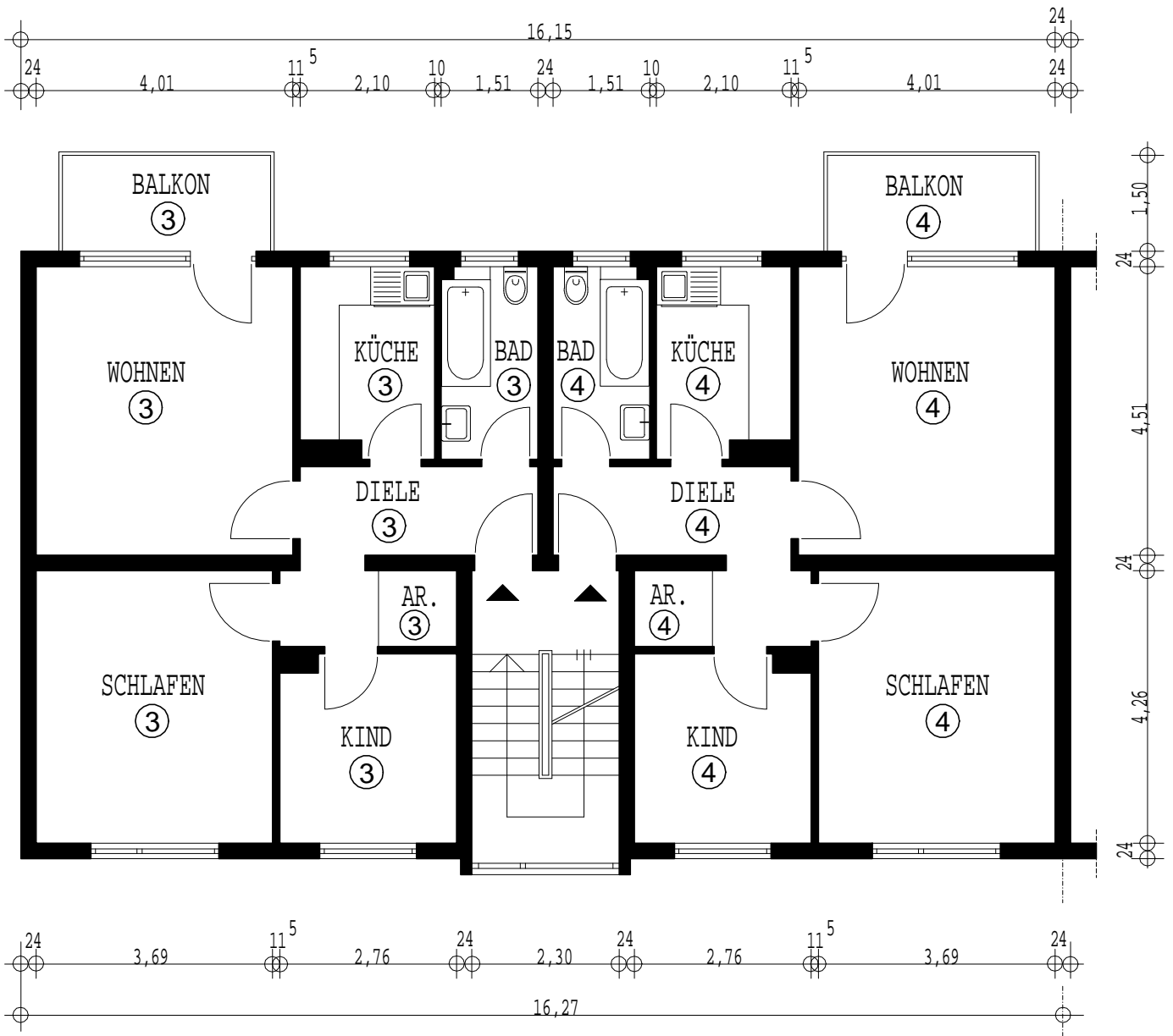
AUFTEILUNGSPLAN GRUNDRISS - BEISPIEL
